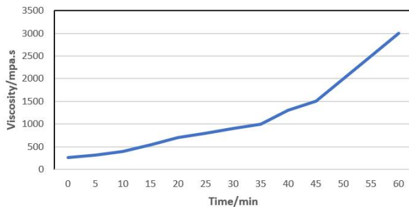
8856A /8856B盘寿命图 (45℃)
