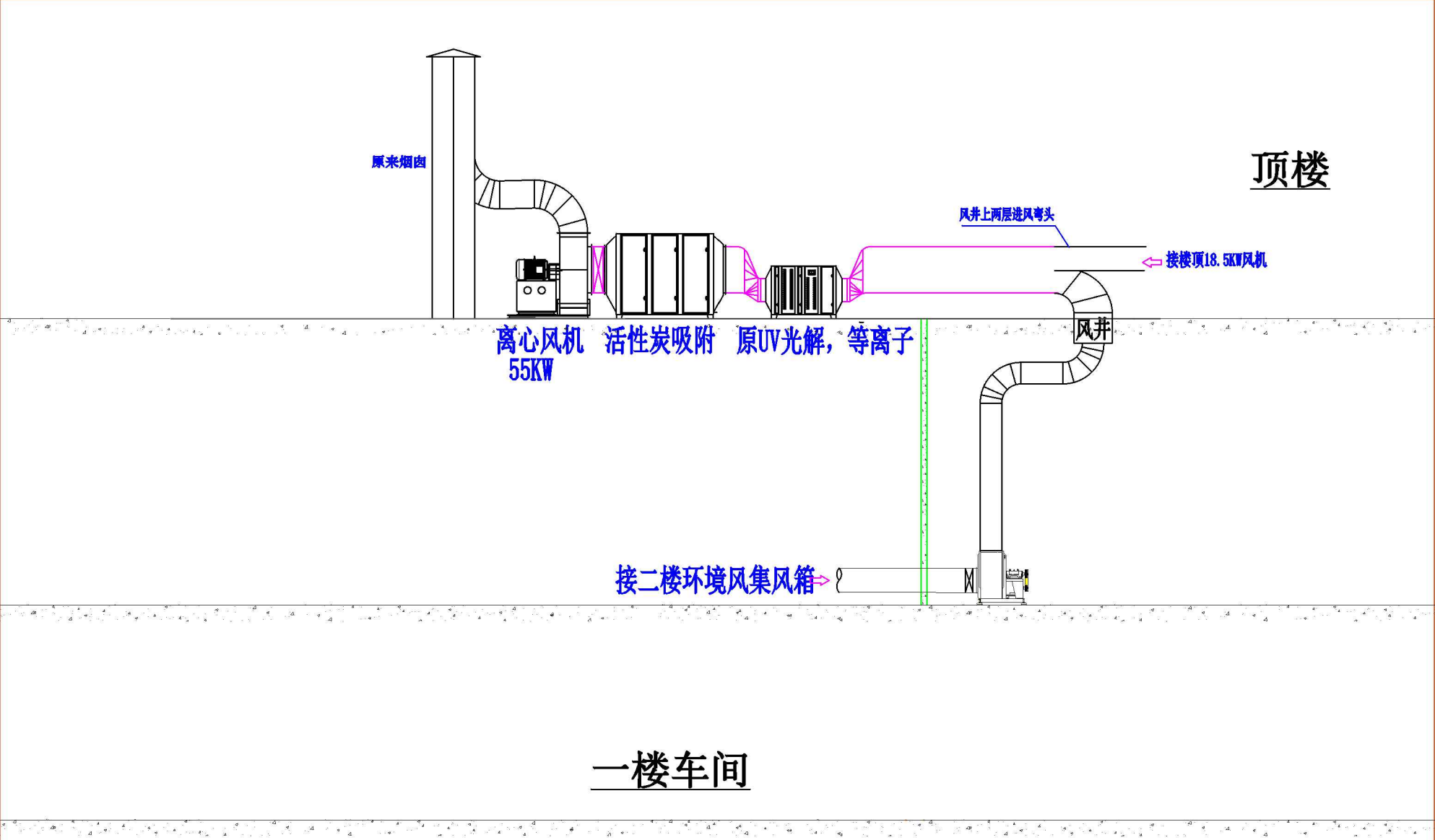
废气处理系统流程示意图
